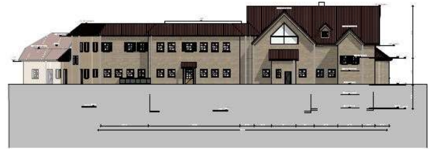
Ansicht West Gastrogebäude M1:200
