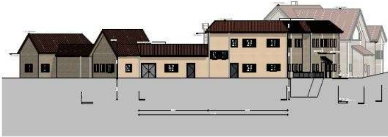
Ansicht Nord Gastrogebäude M1:200
